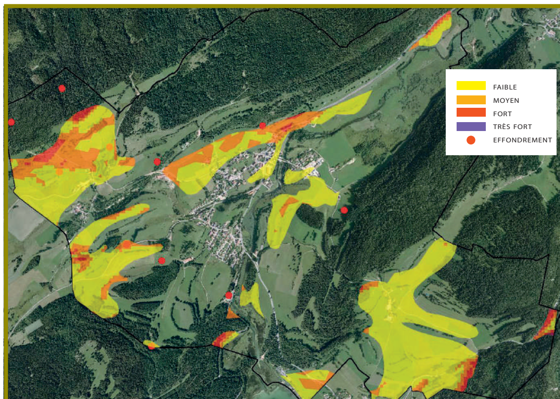
POTENTIEL D'INSTABILITÉ DES TERRAINS (ATLAS DES ZONES À RISQUES DU DÉPARTEMENT DU DOUBS)
